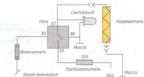
Схема подключения нагревателя к бортовой сети автомобиля.
